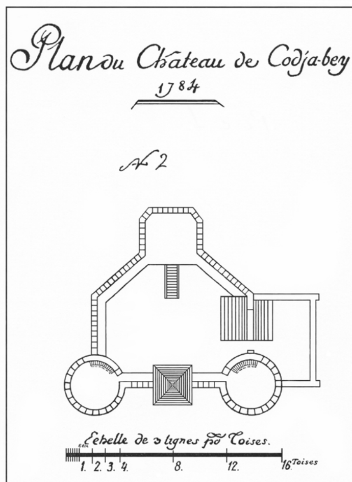
Рис. 6. «План замка Коджа-Бей» 1784 г. (копия 1960-х гг.).
